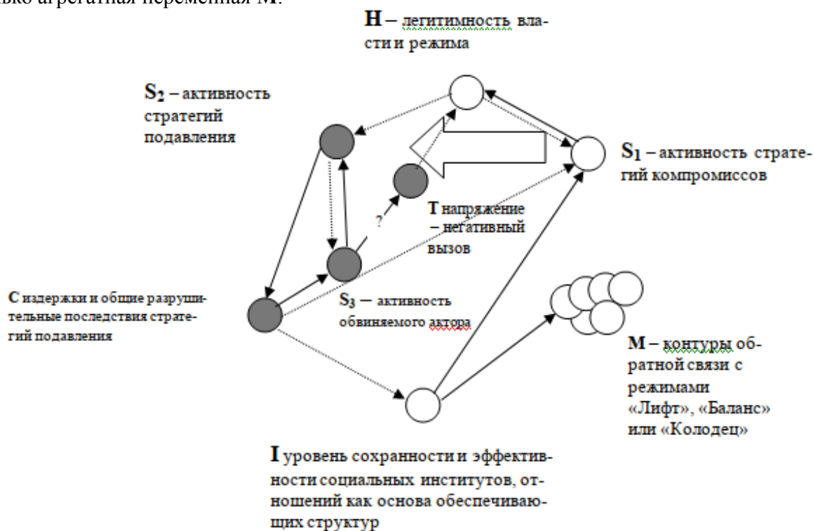
Рис. 4. Издержки C ведут к деградации институтов I , что при эскалации конфликта приводит к системному изменению взаимосвязей агрегатной переменной M : от режима «Баланс» к режиму «Колодец» (паттерн отчуждения).
