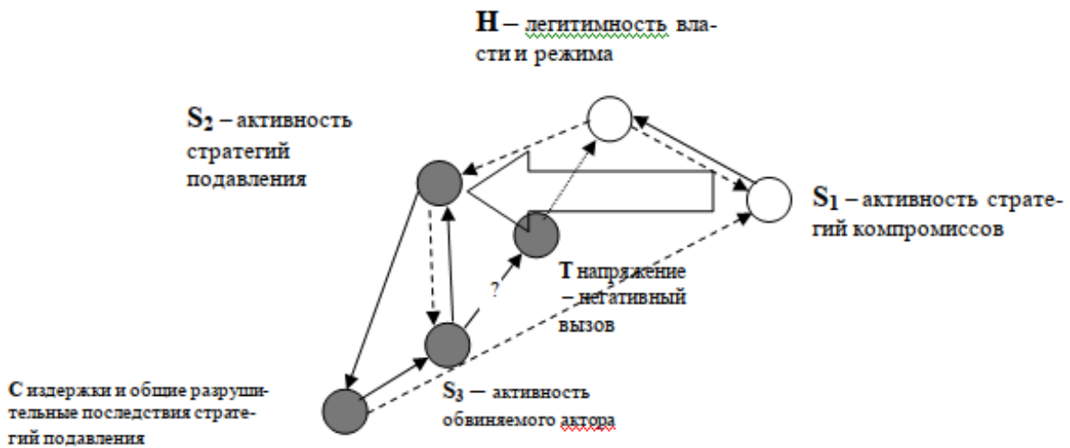
Рис. 3. Переключение ответа на подавление активности обвиняемого актора приводит к эскалации конфликта (контур обратной положительной связи S_2 \rightarrow C \rightarrow S_3 \rightarrow S_2 ) и еще большему ослаблению прежних стратегий переговоров и компромиссов S 1 .
